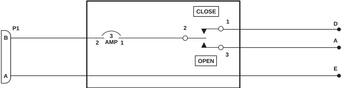
WIRING SCHEMATIC
